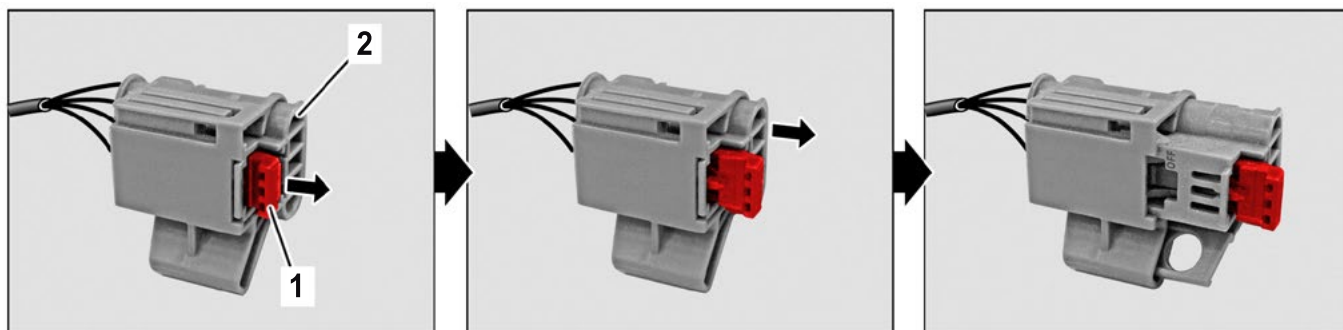
Dispositivo di disinserimento alto voltaggio nel bagagliaio
