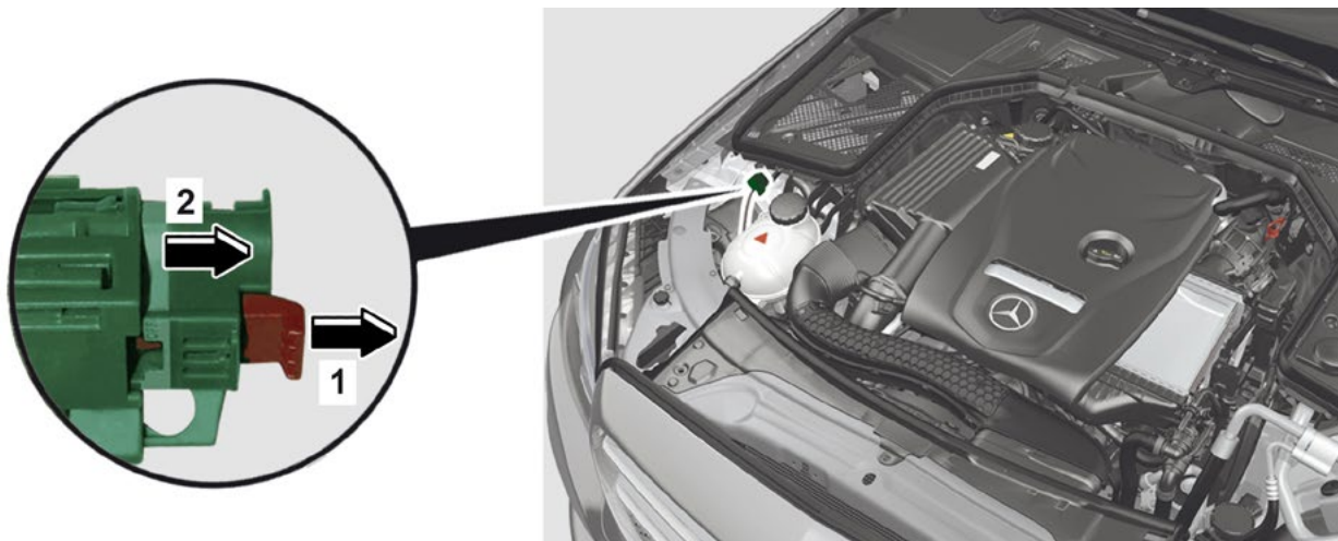
Dispositivo di disinserimento alto voltaggio nel vano motore
